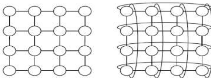
图 3.15 (a)Mesh 拓扑结构 (b)Torus 拓扑结构(宋体, 五号, 居中, 段前段后不空行)
